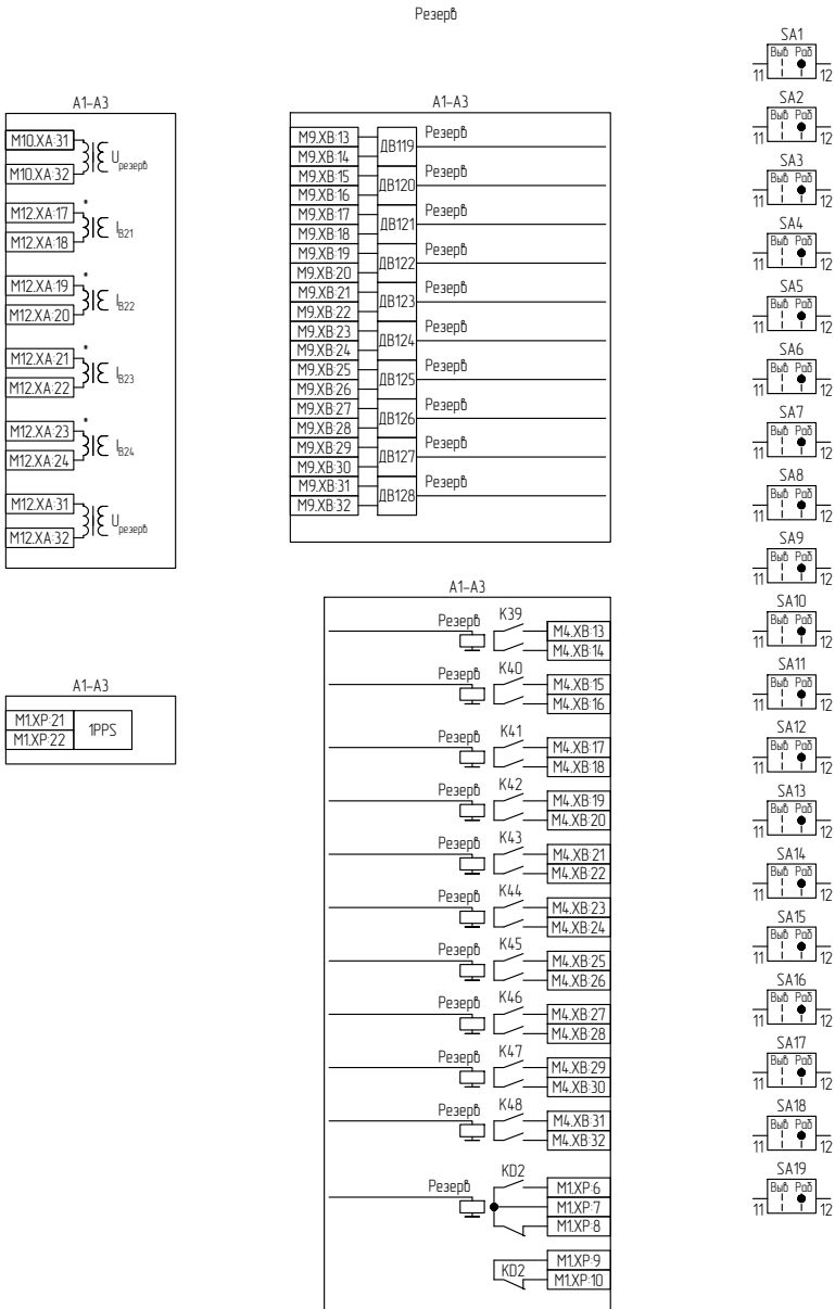
Рисунок Г.19 – Схема электрическая принципиальная (часть 19)
