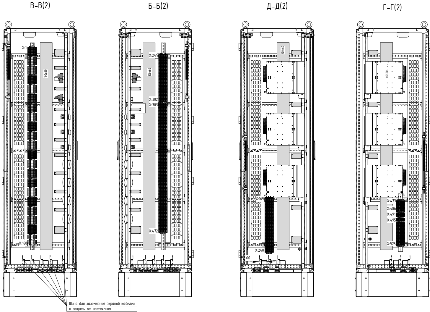
Рисунок В.3 – Чертеж общего вида (часть 3)
