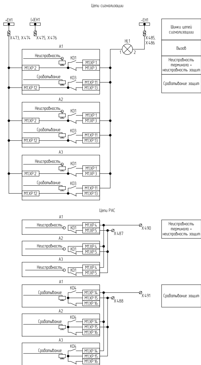
Рисунок Г.18 – Схема электрическая принципиальная (часть 18)
